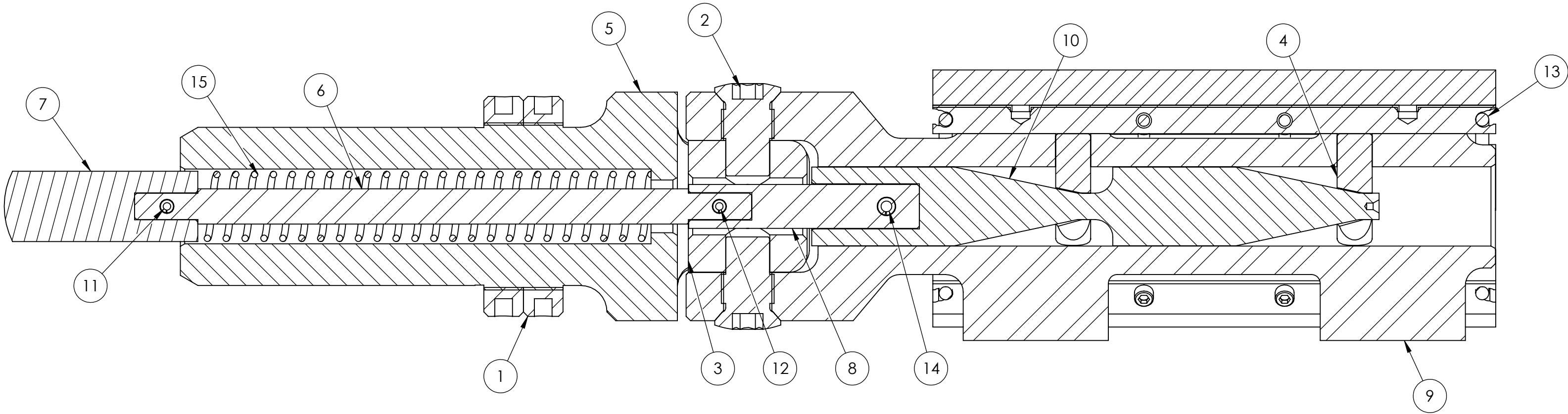
SECTION A-A
