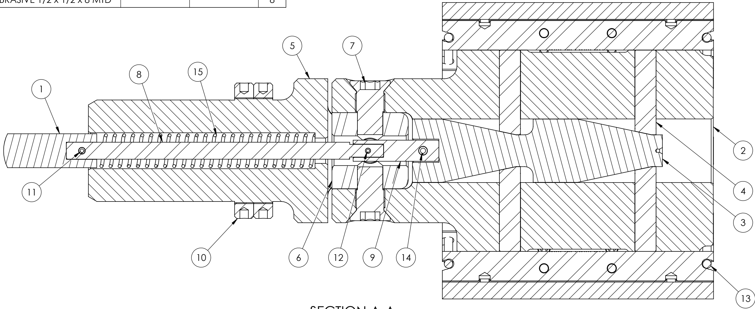
SECTION A-A
